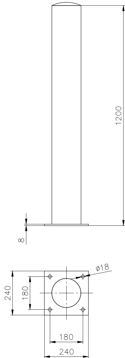
Stahlrohr Ø 159 x 4,5 mm Feuerverzinkt
